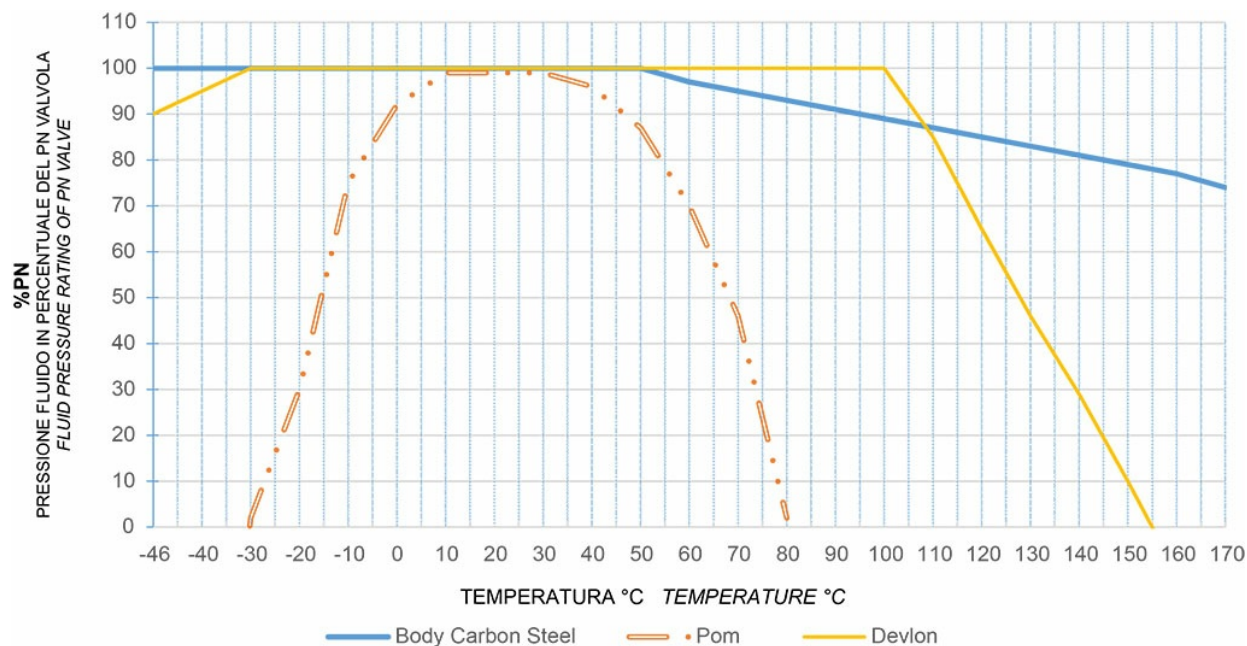
Diagrama de pressão/temperatura
