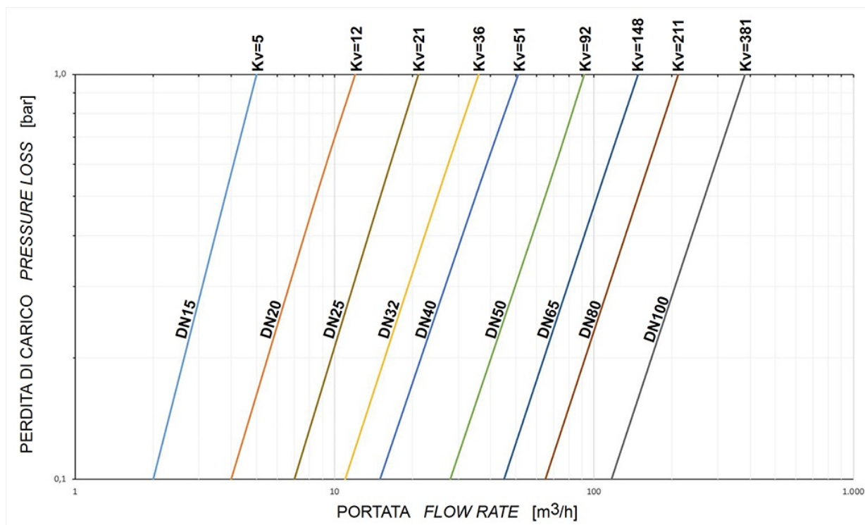
Fluxo/queda de pressão e coeficiente nominal Kv
