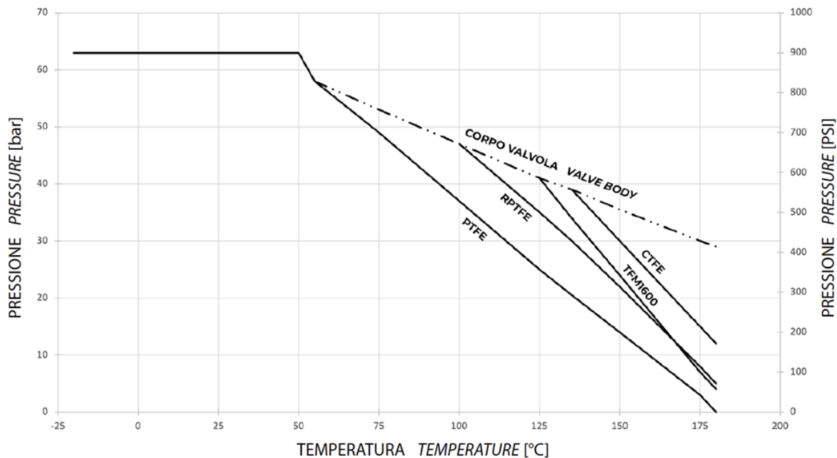
DIAGRAMME PRESSION/TEMPÉRATURE
