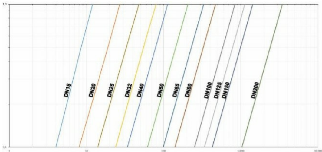
Capacidad de carga/pérdida de carga y coeficiente nominal Kv
