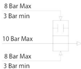
Schema di funzionamento nella configurazione a doppio effetto
