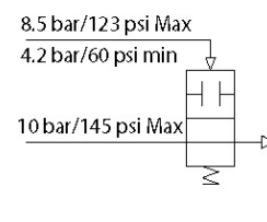
Schema di funzionamento nella configurazione a semplice effetto normalmente aperto Spring return Normally open VIP Working plan
