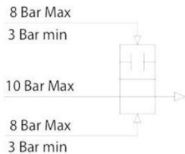
Schema di funzionamento nella configurazione ne doppio effetto
