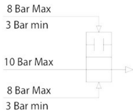
Schema di funzionamento nella configurazione doppio effetto
