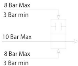
Schema di funzionamento nella configurazione doppio effetto
