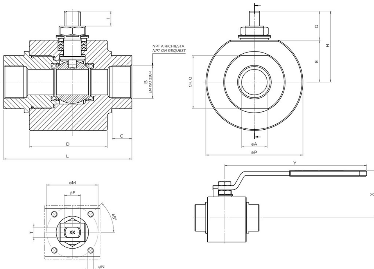
尺寸规格
